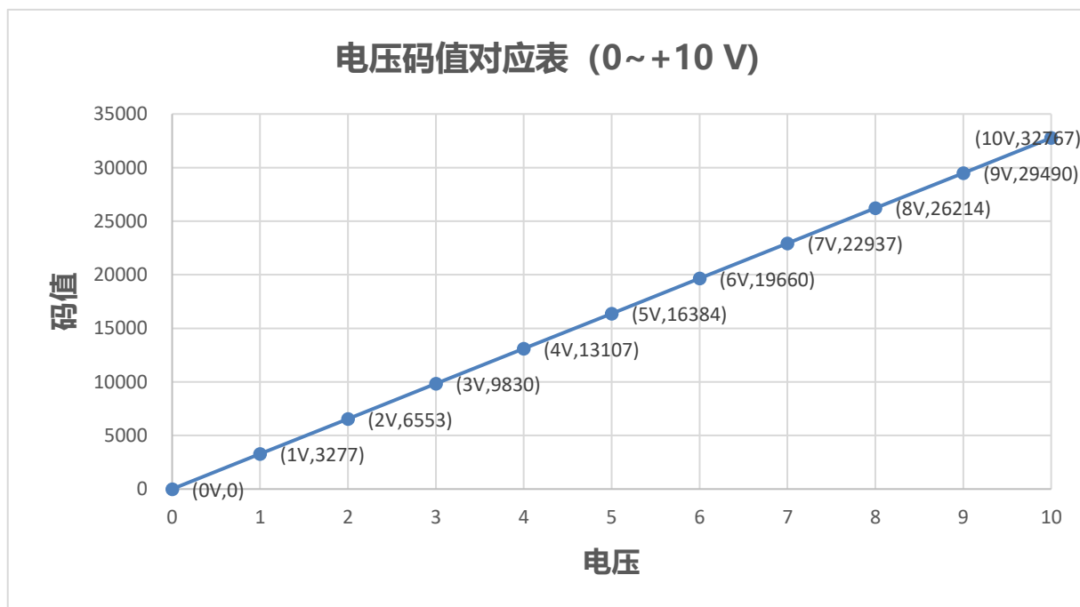
● 表② 0 ~+10 V 码值对应表
