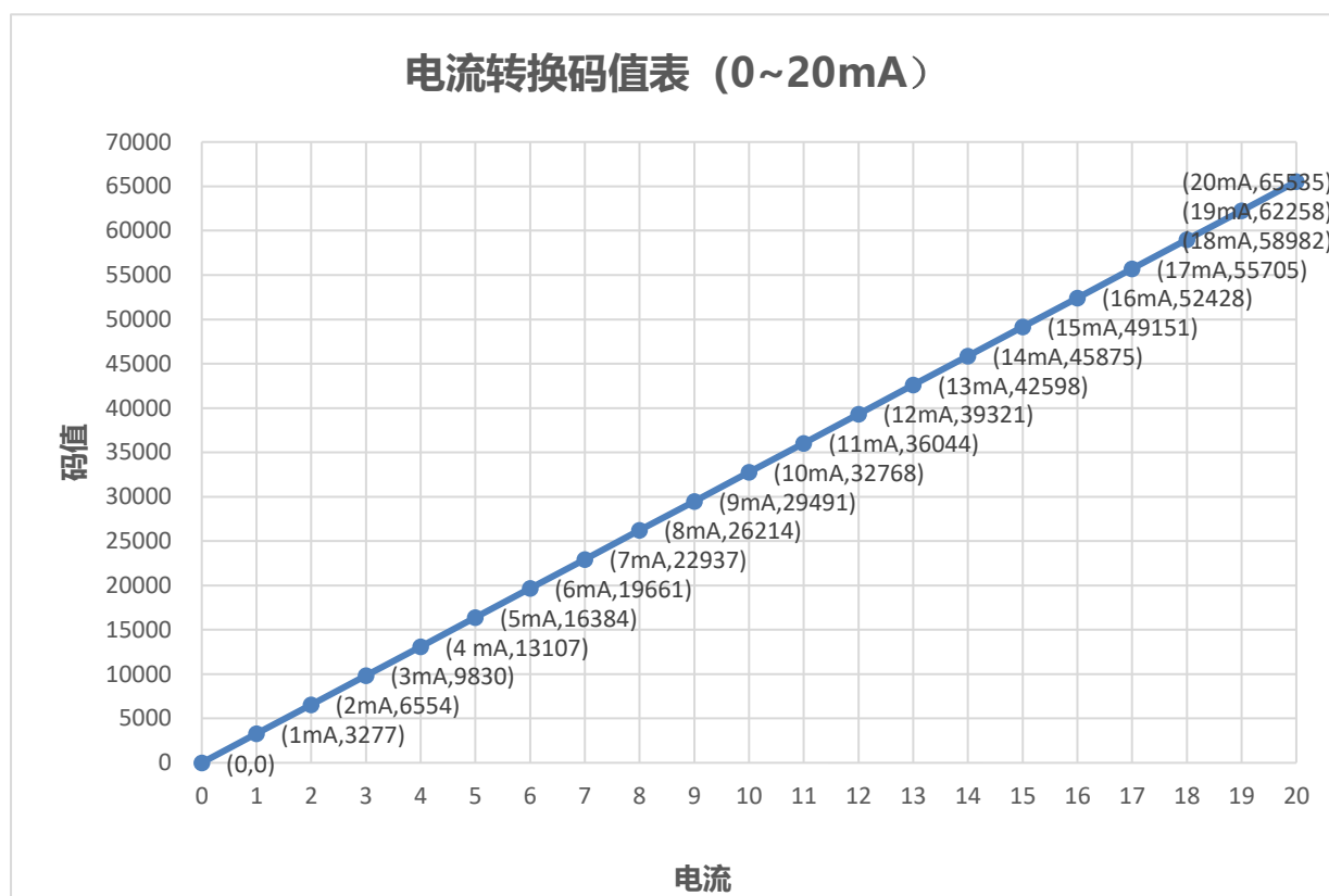
●表④ 0~20 mA 码值对应表
